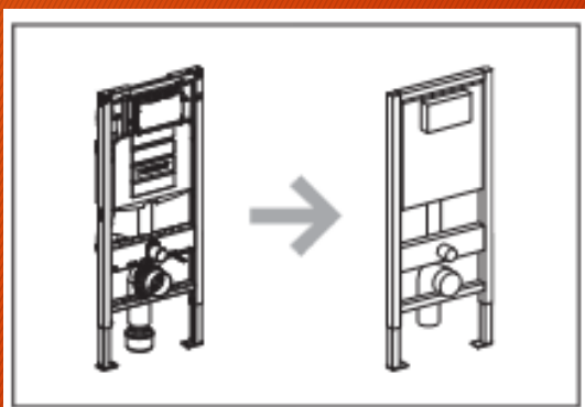
Wandkonstruktion höhenverstellbar
